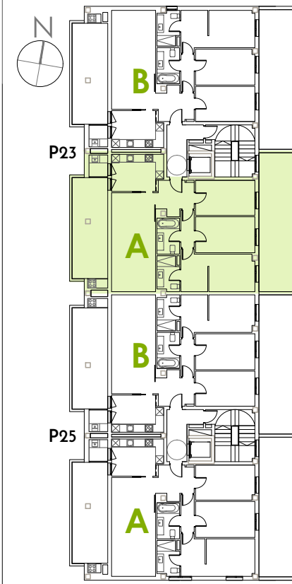
PLANTA 1ª
